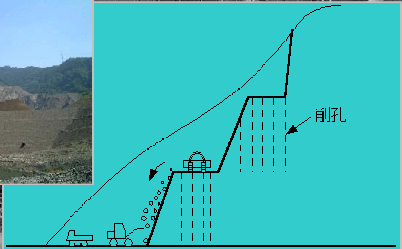
ベンチカット工法
